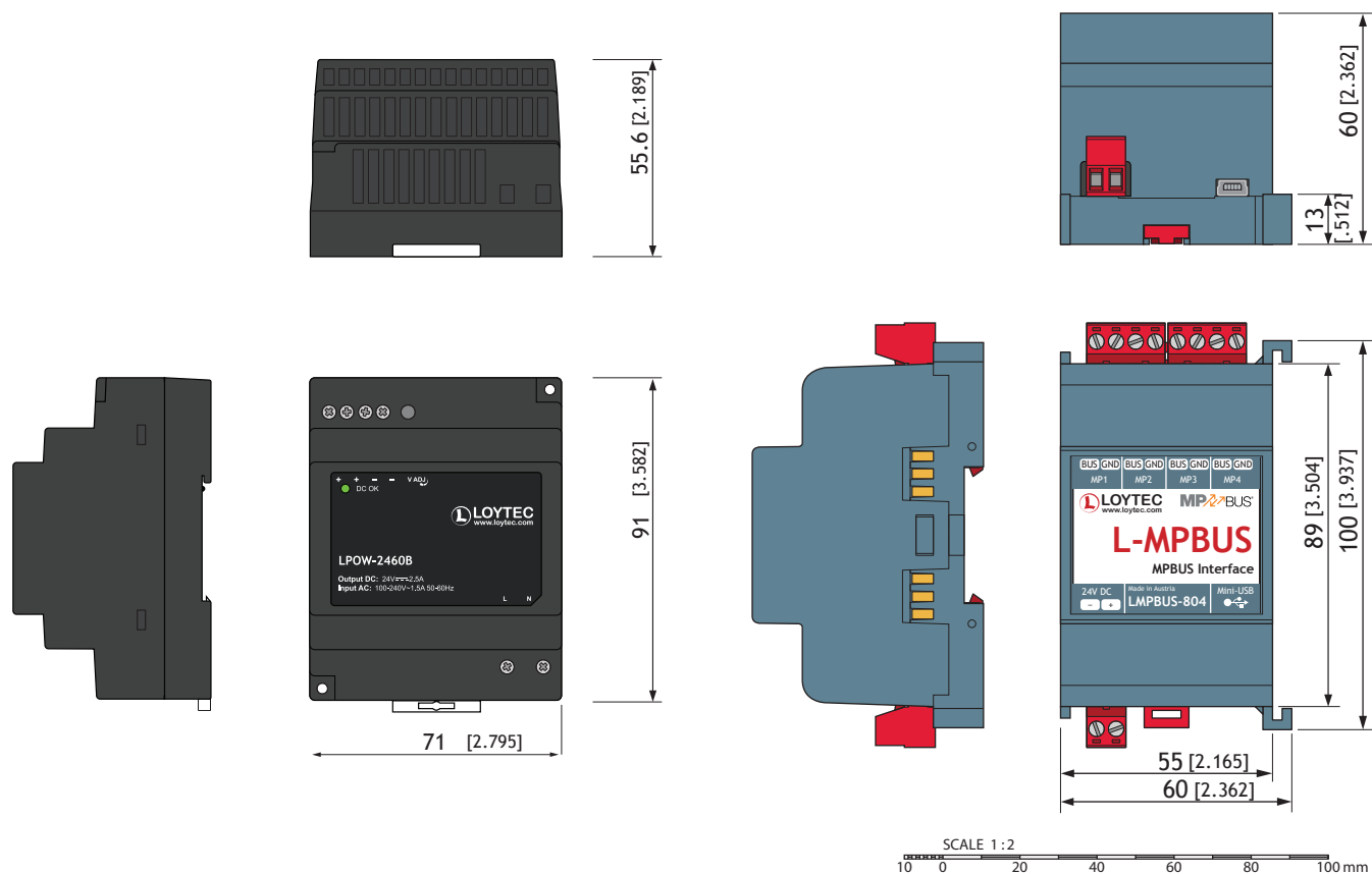
DIM051 LMPBUS-804
