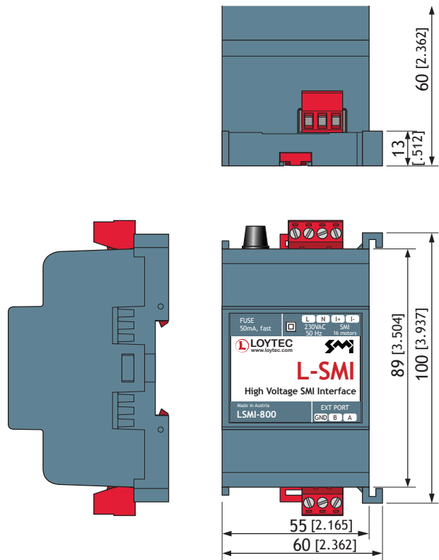
DIM033 LSMI-800
